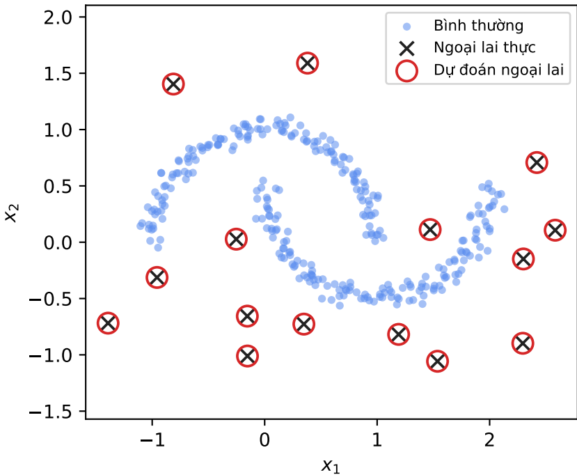
LOF — k=20
